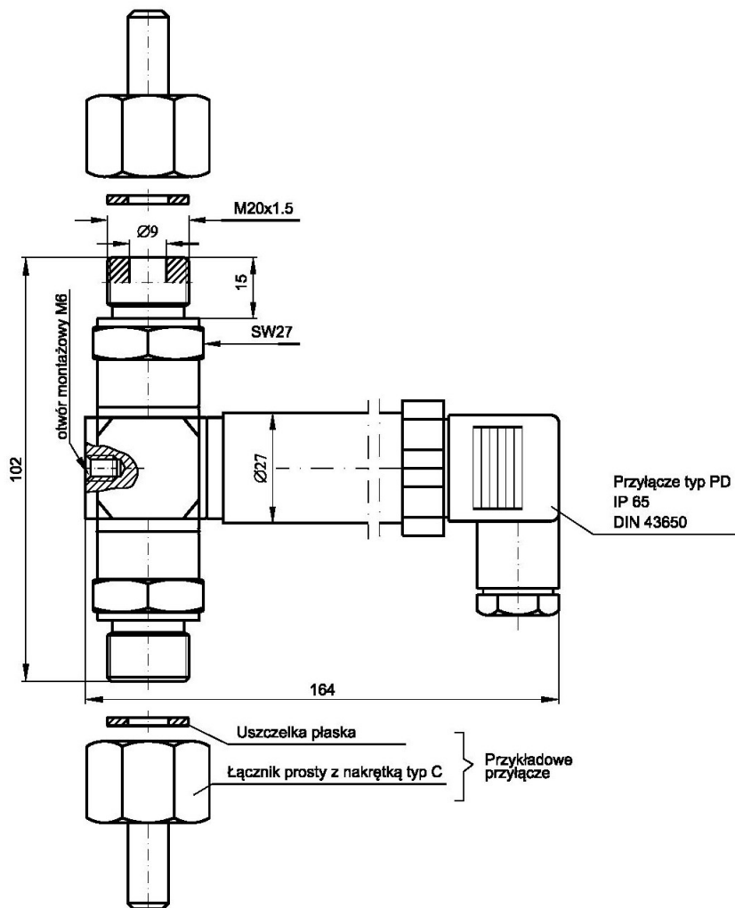
Rys.9. Przetwornik różnicy ciśnień serii PR-28 Safety. Gabaryty.
