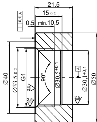
Rys.8f. Pierścień do współpracy z przyłączem typu CG1 z membraną czołową Materiał – stal 00H17N14M2 Kod zam. Gniazdo CG1
