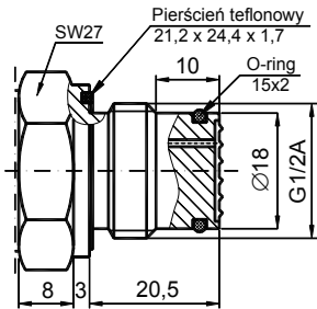
Rys.8c. Przyłącze z czołową membraną typu CG1/2 z gwintem G1/2"
