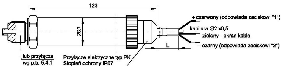
Rys.3b. Przetwornik PC-28 Safety z przyłączem PK.
