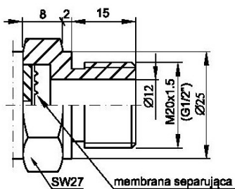
Rys.6a. Przyłącze typu P z gwintem M20x1,5 z powiększonym otworem \varnothing 12
