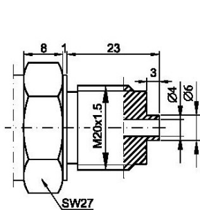
Rys.5a. Przyłącze manometryczne typu M z gwintem M20x1,5
