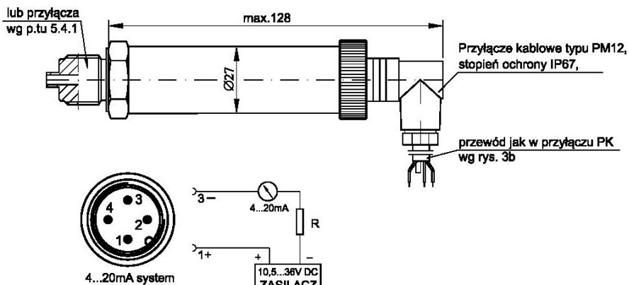
Rys.3d. Przetwornik PC-28 Safety z przyłączem PM12
