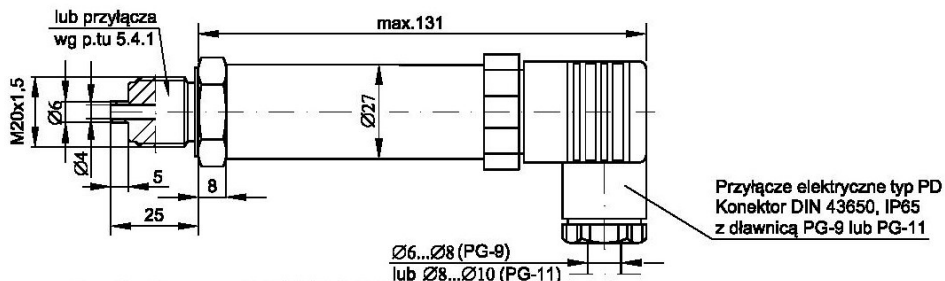
Rys.3a. Przetwornik PC-28 Safety z przyłączem PD.
