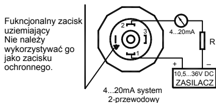
Rys.2. Schemat połączeń elektrycznych przetworników z przyłączem PD (nie dotyczy wyk. Ex)
