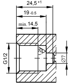
Rys.8b. Gniazdo do współpracy z przetwornikami z przyłączem typu G1/2
