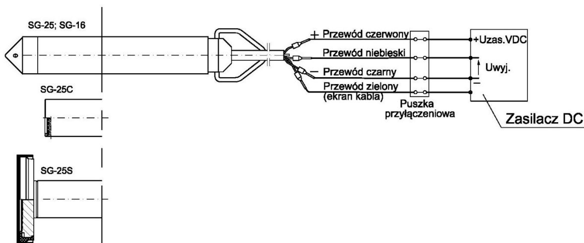
Rysunek 4. Podłączenie elektryczne sondy w wykonaniu trójprzewodowym, wyjście napięciowe.
