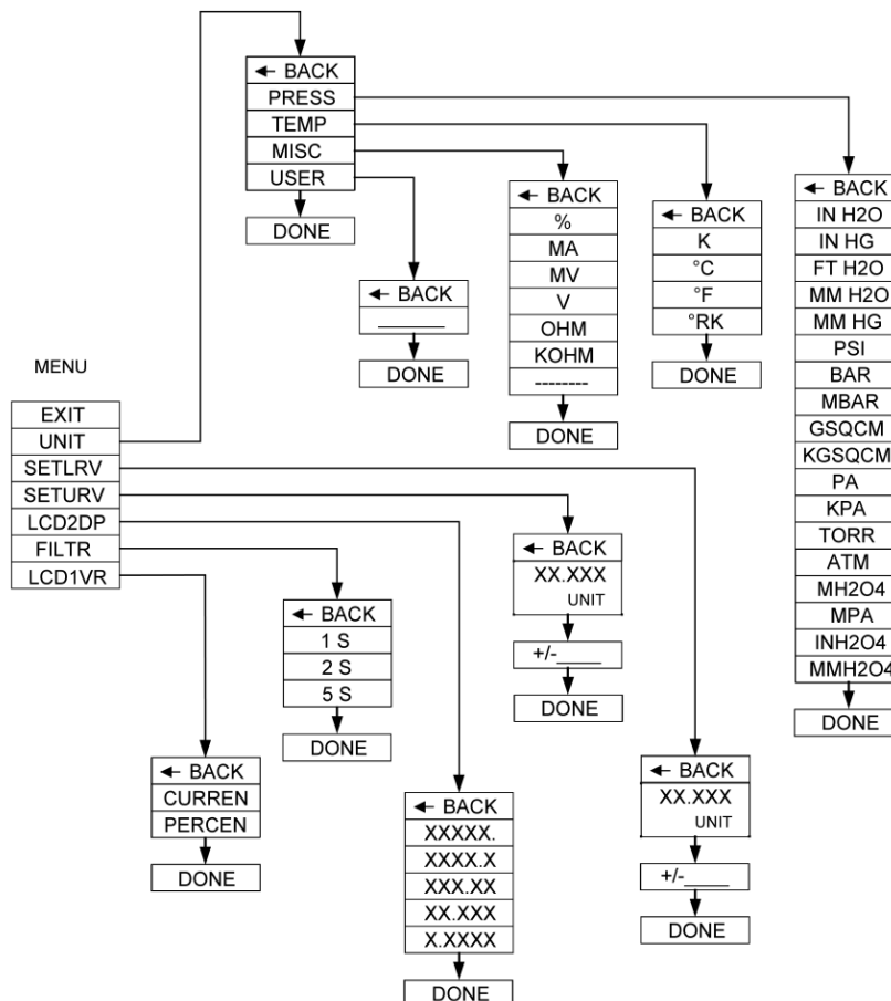
Rysunek 5. Struktura MENU lokalnych nastaw
