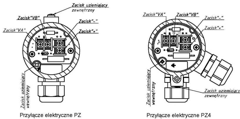
Rys. I.5. Przyłącze typu PZ i PZ4.
