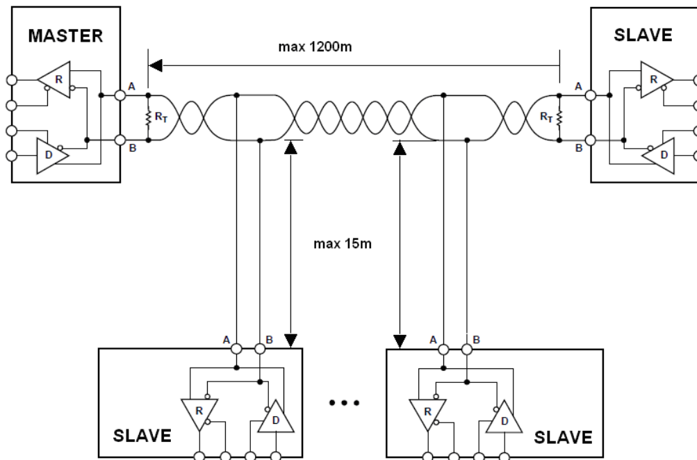
Rysunek 2. Przykład konfiguracji sieci Modbus
