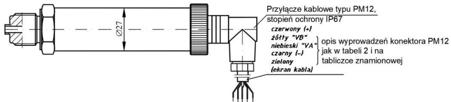
Rys. I.4. Przyłącze typu PM12.
