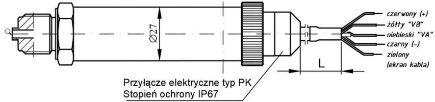
Rys. I.1. Przyłącze typu PK.
