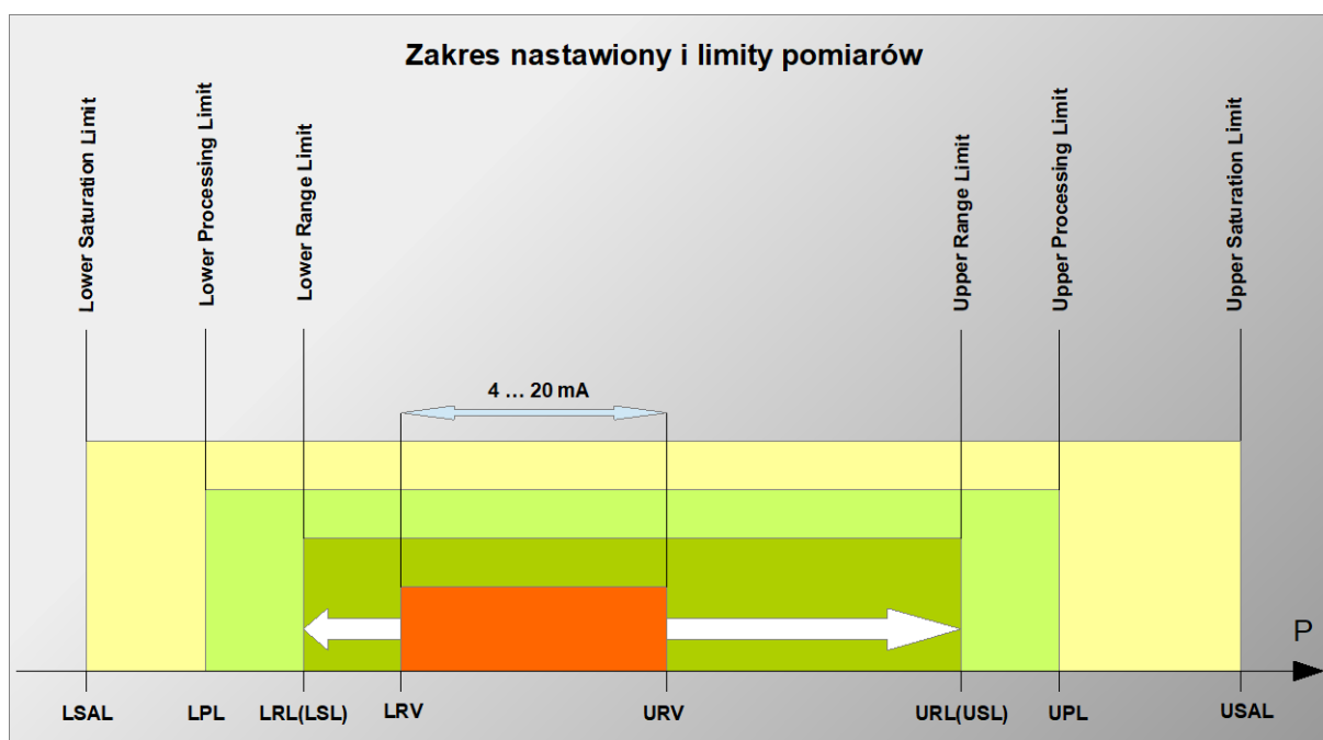
Rysunek 3. Zakres nastawiony i limity pomiarów
