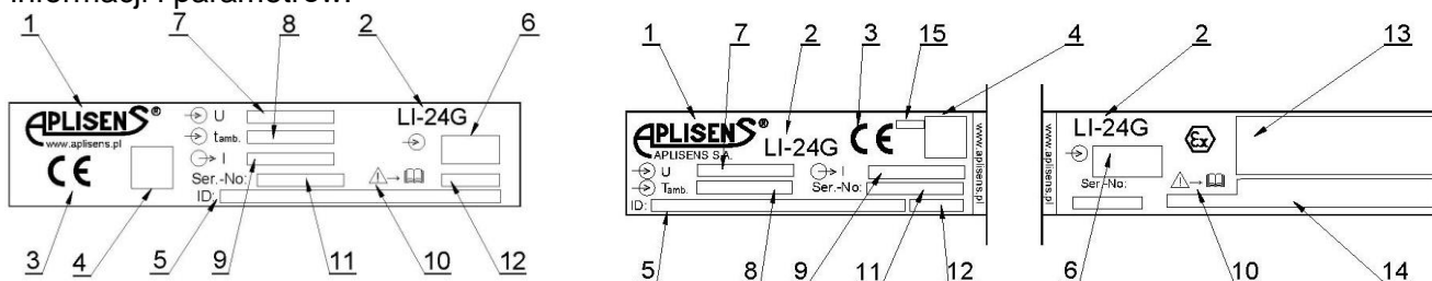
Rysunek 3. Przykładowe tabliczki znamionowe LI-24G w wykonaniu standardowym i Exi.
