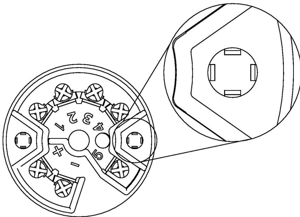
Rysunek 7. Blokada przeciw wypadaniu wkrętów mocujących w przetworniku LI-24G.
