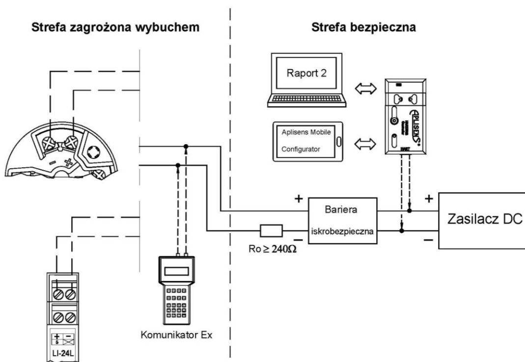
Rysunek 12. Podłączenie elektryczne 4...20 mA HART do przetworników w wykonaniu Exi.
