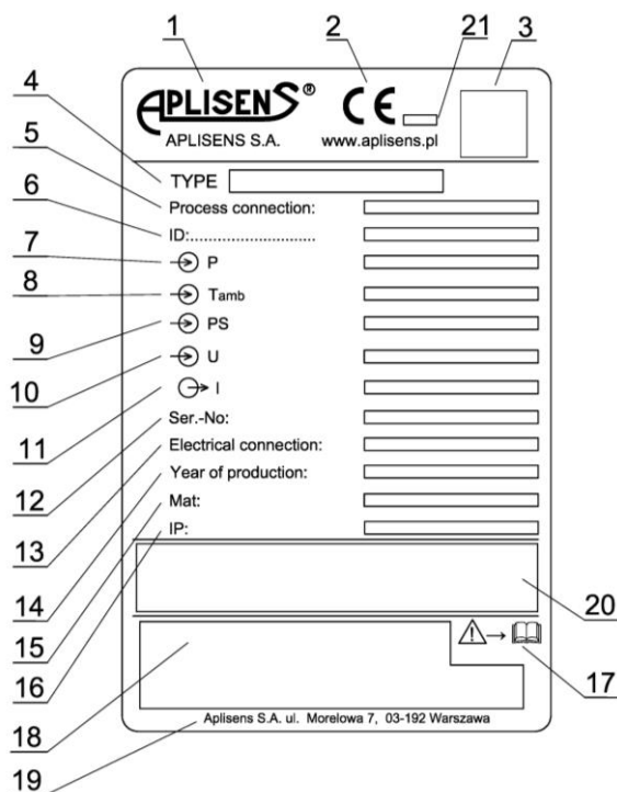
Rysunek 2. Przykładowa tabliczka znamionowa.
