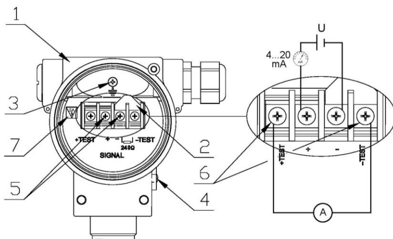
Rysunek 7. Podłączenie elektryczne przetwornika.
