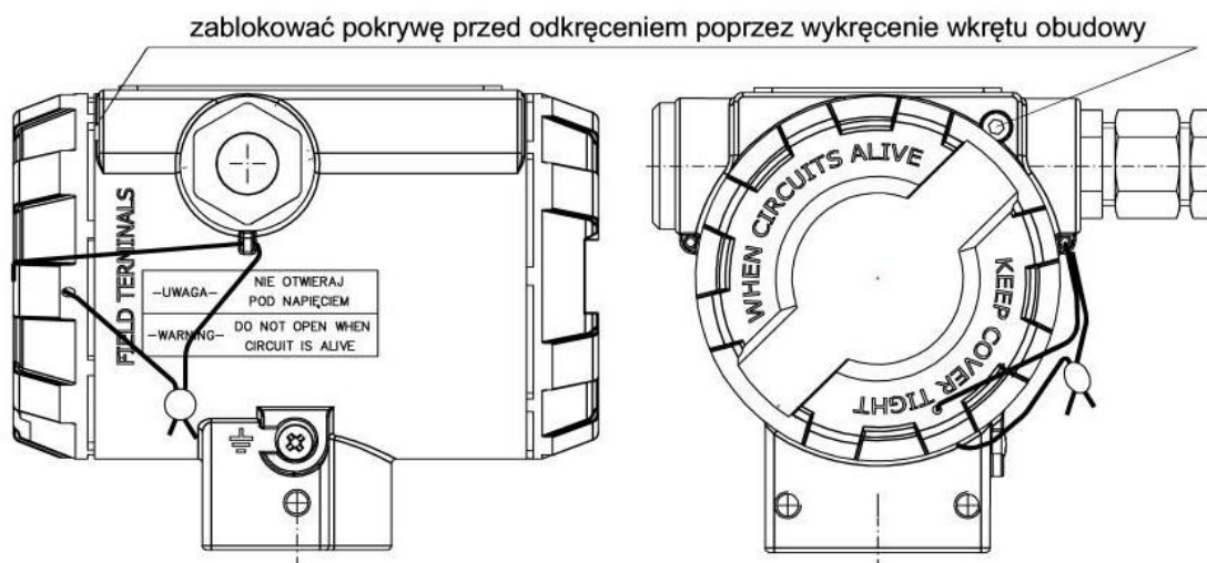
Rysunek 6. Sposób plombowania przetworników.
