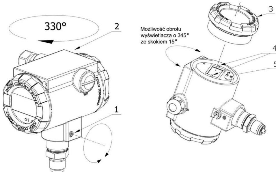
Rysunek 11. Obrót obudowy, zmiana pozycji wyświetlacza oraz dostęp do przycisków.
