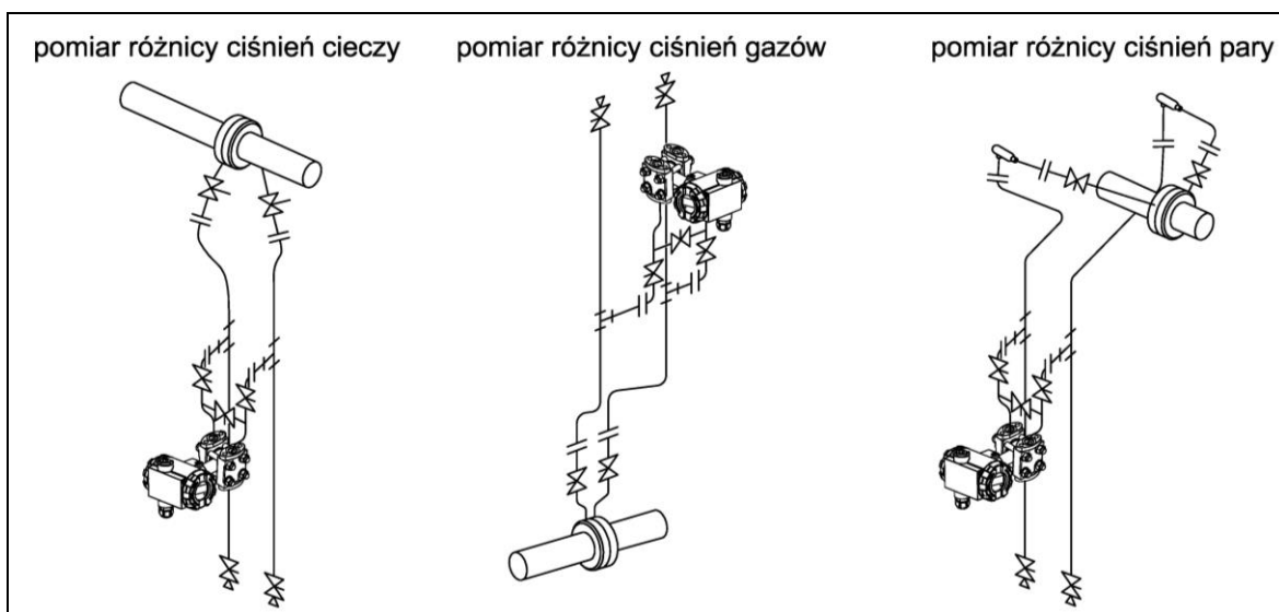
Rysunek 4. Przykłady montażu przetworników różnicy ciśnień.
