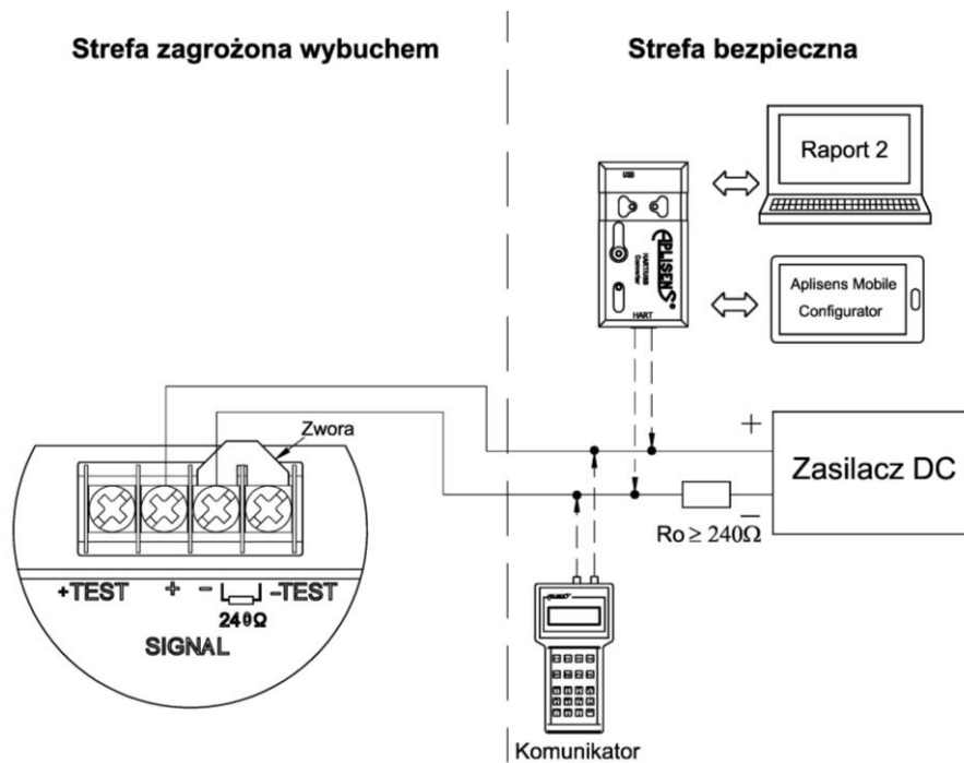
Rysunek 9. Podłączenie elektryczne 4...20 mA HART do przetwornika w wykonaniu Exd.
