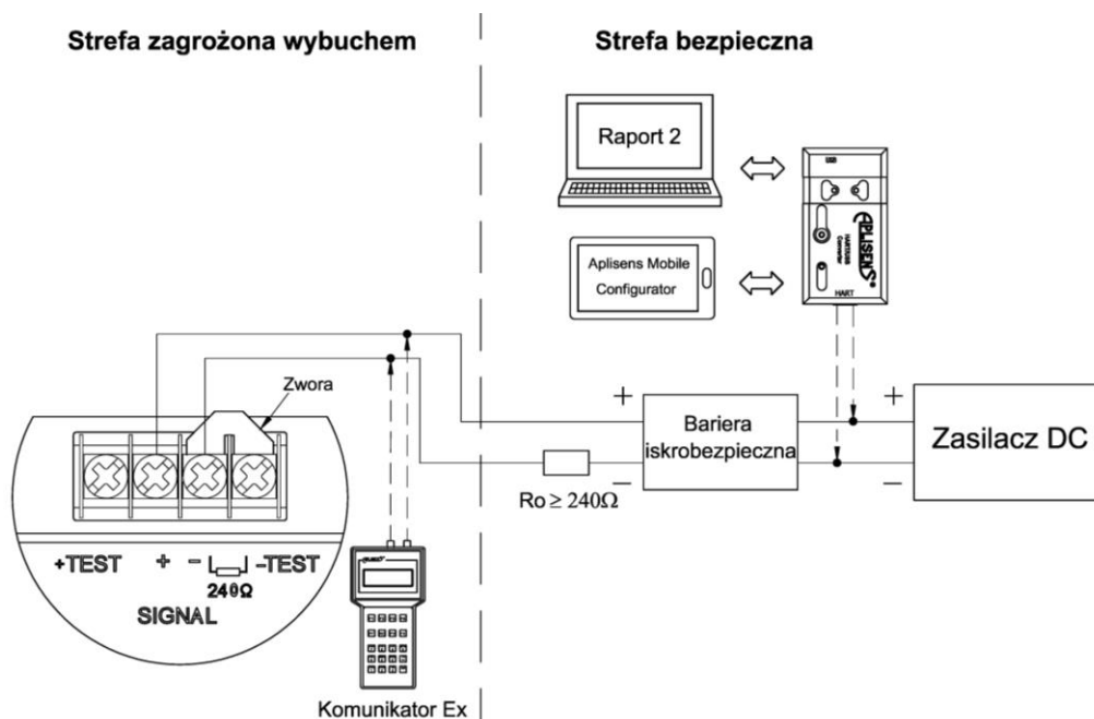
Rysunek 10. Podłączenie elektryczne 4...20 mA HART do przetwornika w wykonaniu Exi.
