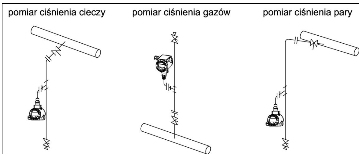
Rysunek 3. Przykłady montażu przetworników ciśnienia.
