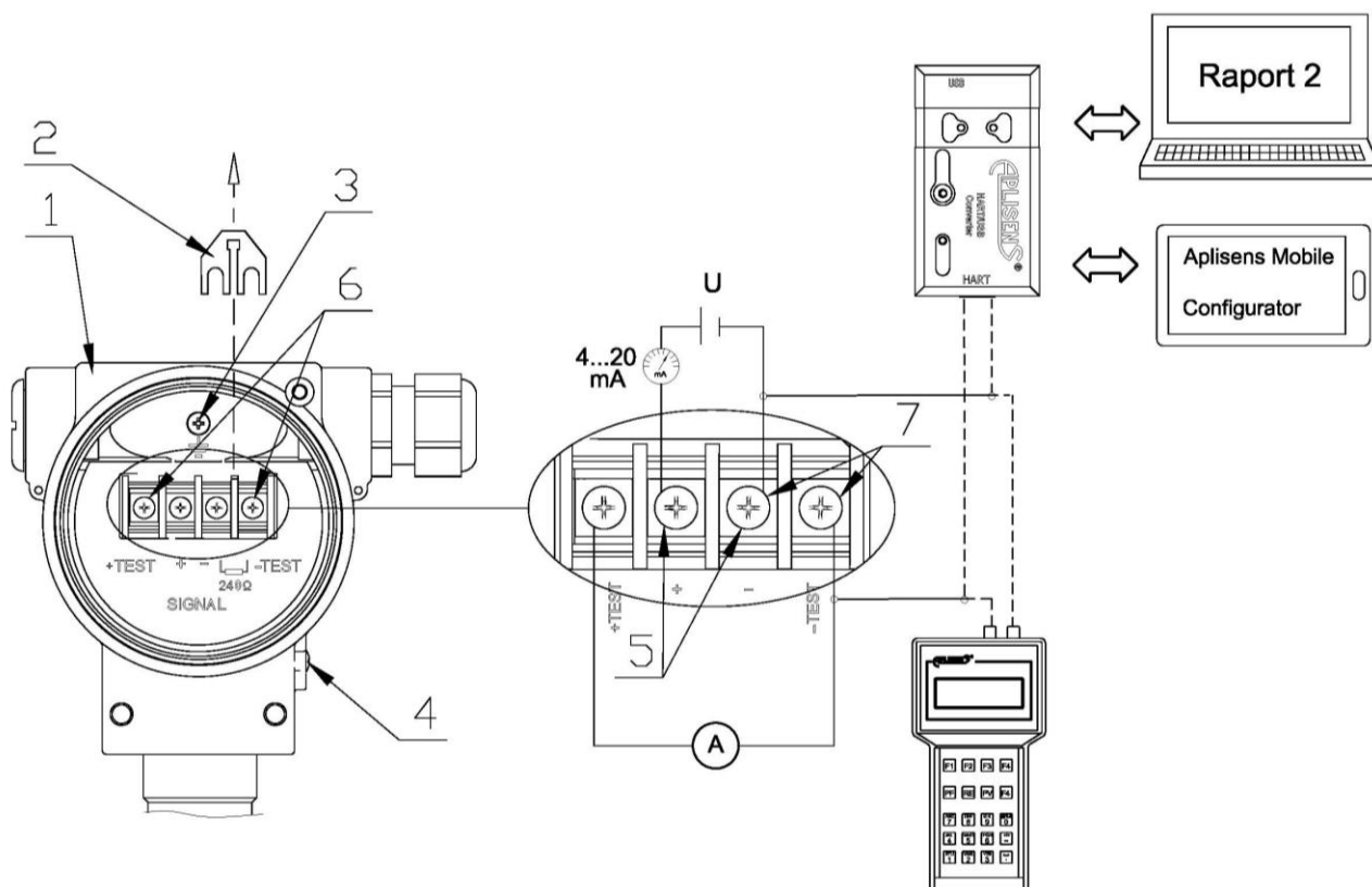
Rysunek 8. Podłączenie elektryczne 4...20 mA HART do przetwornika w wykonaniu standardowym.
