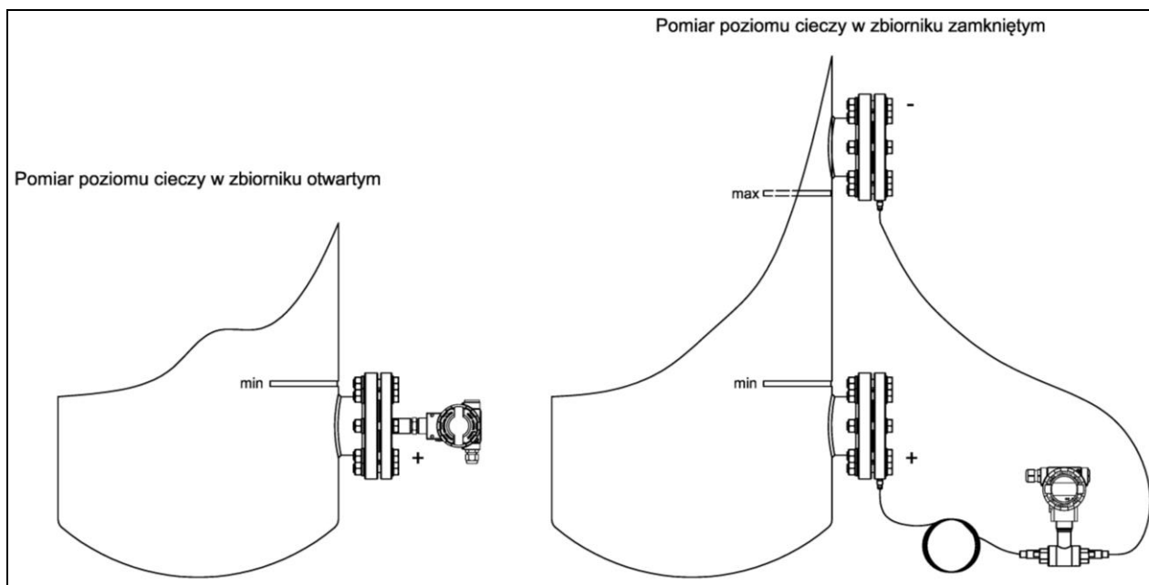
Rysunek 5. Przykłady montażu przetworników na zbiornikach.
